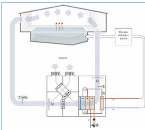
Figura 9. Esquema del sistema de climatización de las piscinas e imagen de una de las máquinas climatizadoras.
